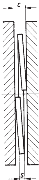
Bild 6. Prüfung der Schränkung
