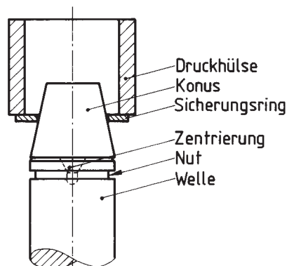
Bild 14. Montage mit Konen
