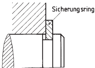
Bild 7. Anlage scharfkantig
