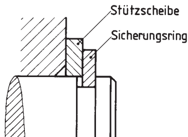
Bild 9. Scharfkantige Anlage am Sicherungsring mit Hilfe einer Stützscheibe
