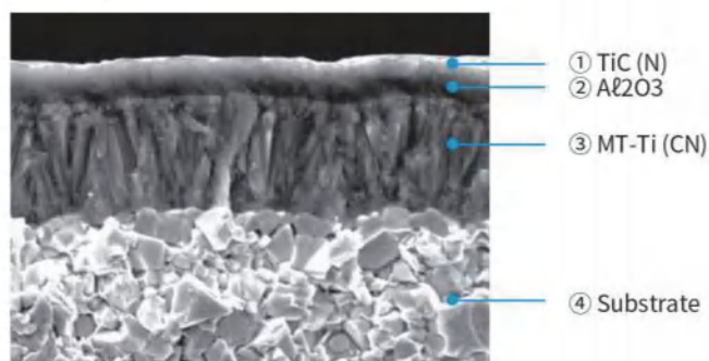
Вид поперечного сечения CVD покрытия Cross-sectional view of CVD coating
