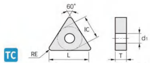
Габаритные размеры (мм) / Dimensions (mm)
