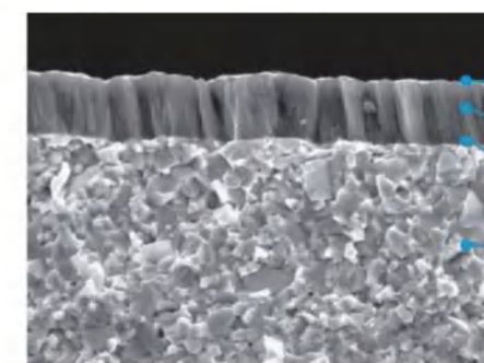
Вид поперечного сечения PVD покрытия Cross-sectional view of PVD coating
