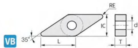
Габаритные размеры (мм) / Dimensions (mm)
